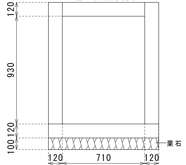
マンホール基礎 北・西立面図
