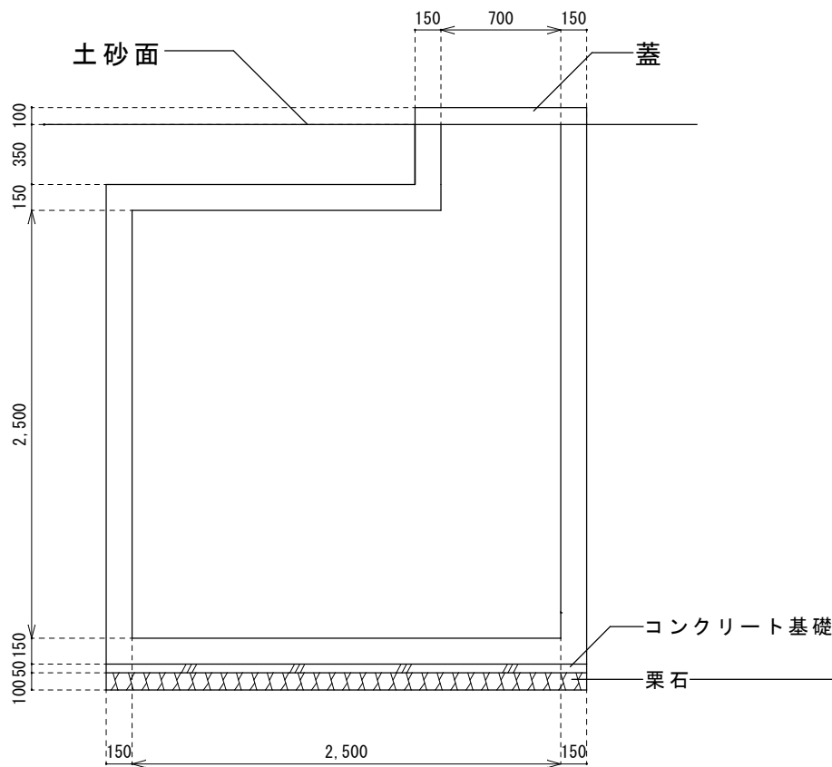
西立面図
